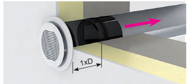
Régulateur RDR BP en extraction
